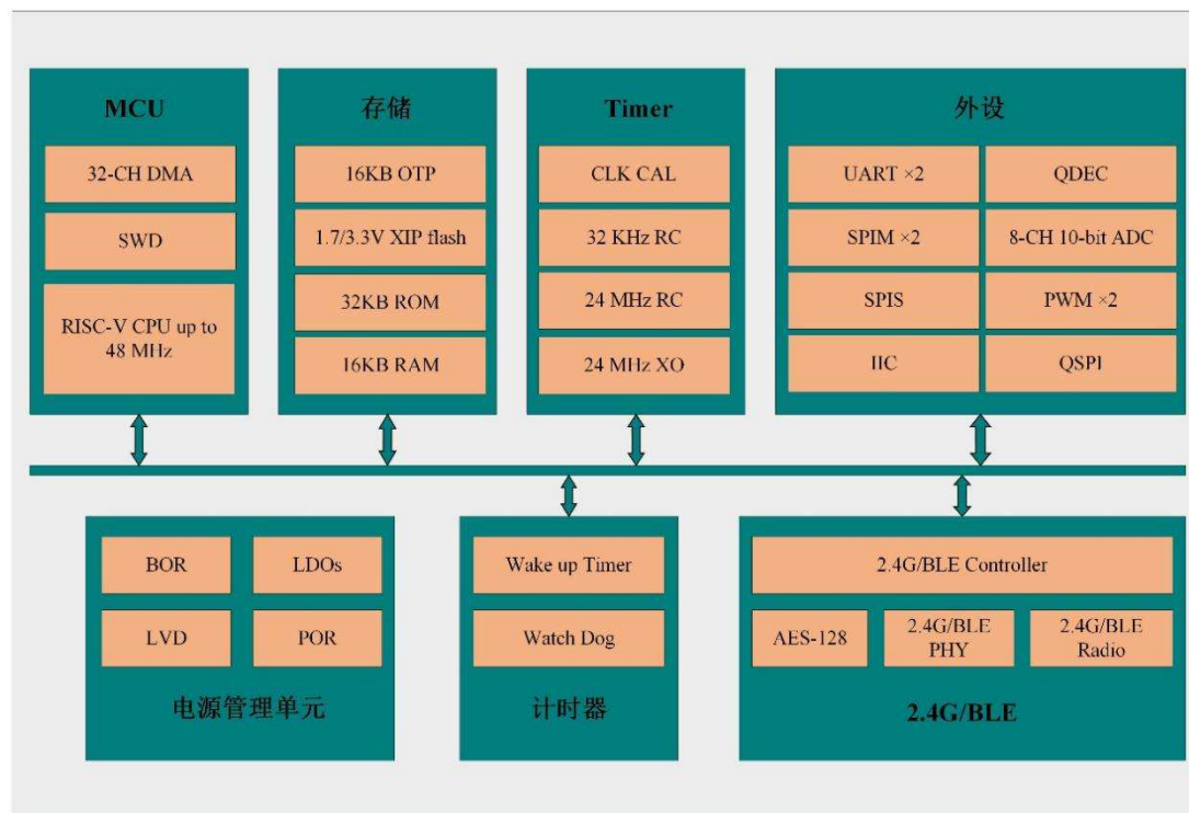
Figure 1-1 系统框图
