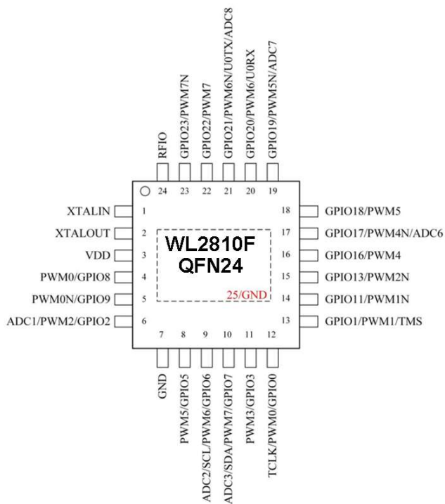
Figure 1-3 QFN24 封装图（底衬为 GND）
