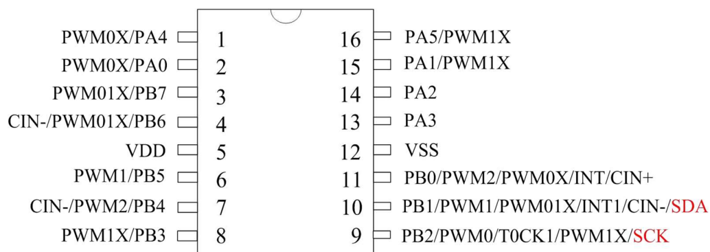
图 3.1 管脚信息（16PIN）
