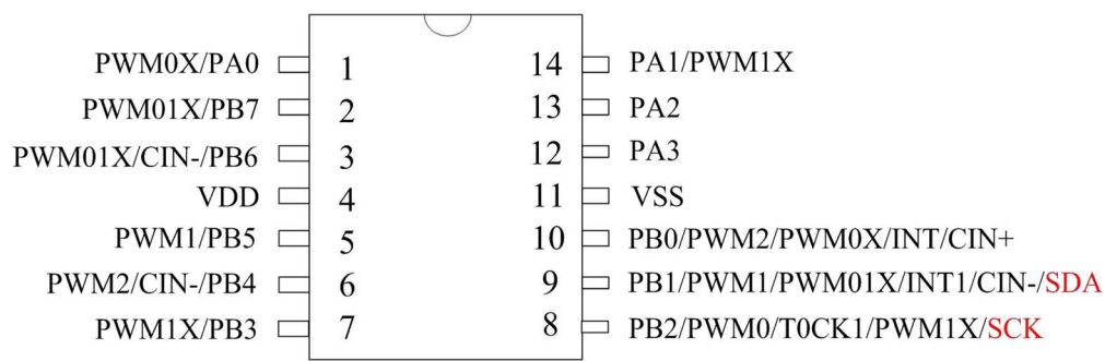
图 3.3 管脚信息（14PIN）
