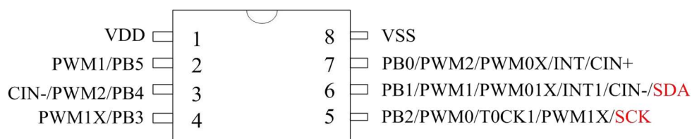
图 3.2 管脚信息（8PIN）
